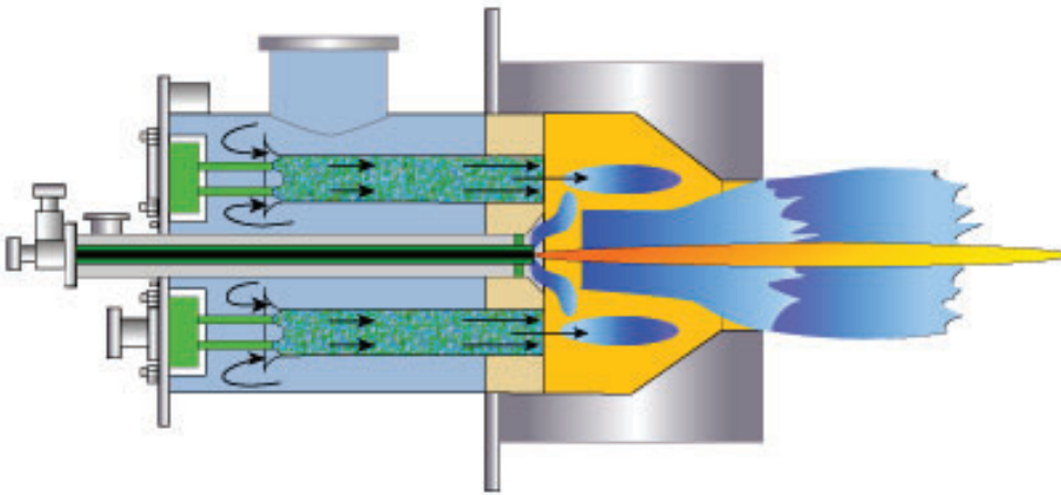
EcoFornax™ LE Burner
